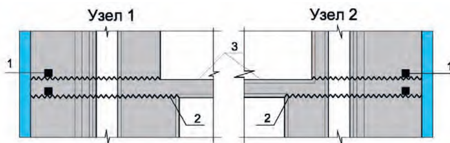
Рисунок 7.1.8 – Типовые узлы гидроизоляции в машинном зале и технологических помещениях (узлы 1 и 2 на рис. 7.1.7): 1 – гидроизоляционный жгут «Пенебар» и «Скоба крепежная металлическая»; 2 – шов бетонирования; 3 – железобетонное перекрытие
