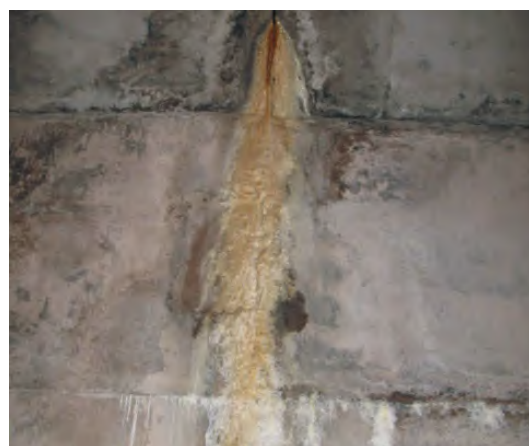
Рисунок 6.7.2 – Транспортно-кабельный туннель: а – выходной оголовок туннеля; б – фильтрация воды через стены туннеля с выносом свободной извести и продуктов коррозии арматуры
