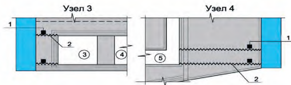
Рисунок 7.1.10 – Типовые узлы гидроизоляции в потернах, цементационных галереях и соединительных коридорах (узлы 3 и 4 на рис. 7.1.9): 1 – гидроизоляционный жгут «Пенебар» и «Скоба крепежная металлическая»; 2 – шов бетонирования; 3 – цементационная галерея; 4 – дренажная галерея (потерна); 5 – соединительный коридор
