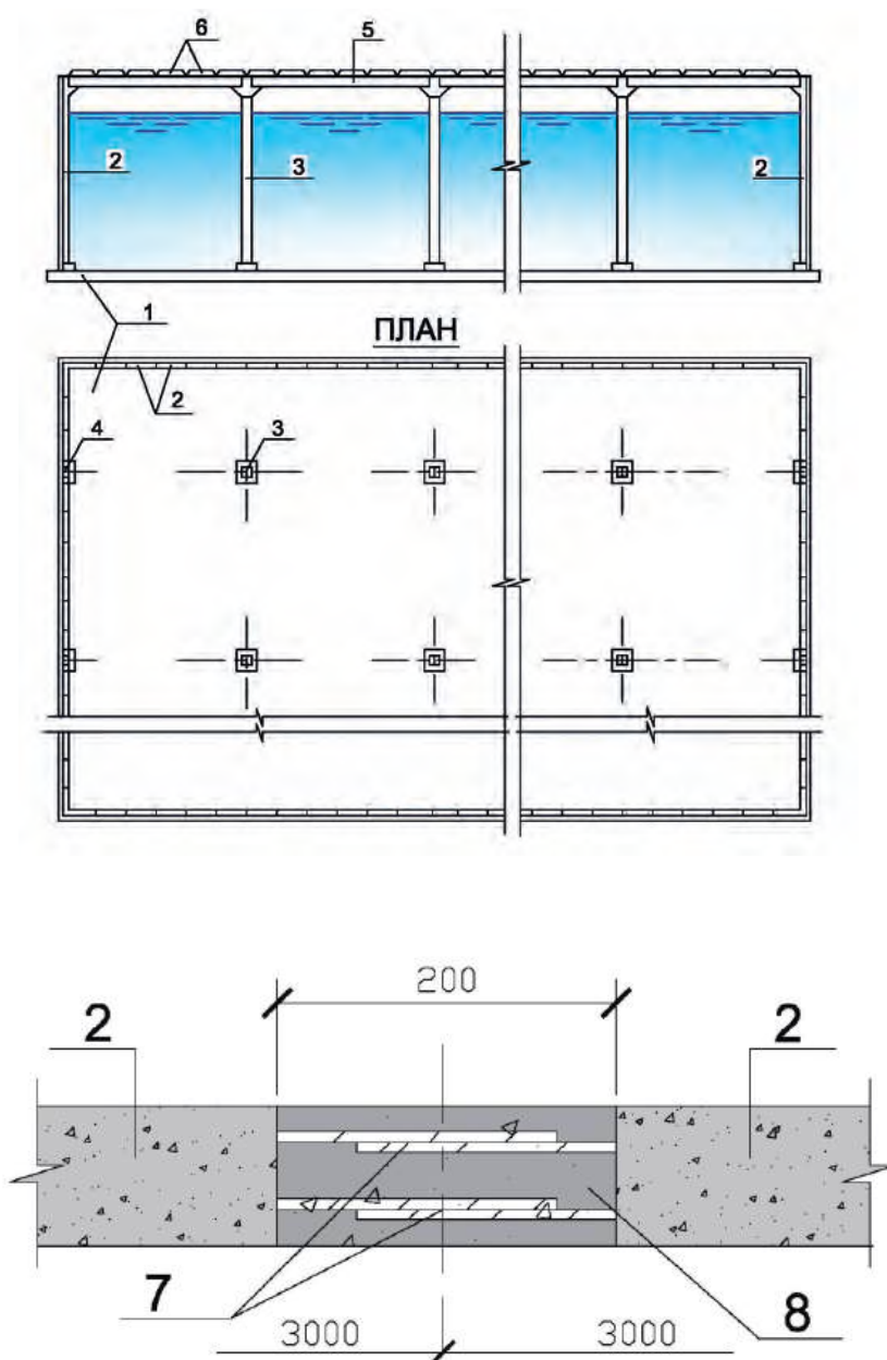
Рисунок 6.4.2 – Схема прямоугольного резервуара из сборных железобетонных панелей: 1 – монолитное днище; 2 – стеновые панели; 3 – промежуточная колонна; 4 – крайняя колонна; 5 – ригель; 6 – плиты перекрытия; 7 – сварка стыков арматуры; 8 – бетон, предназначенный для заполнения швов между панелями
